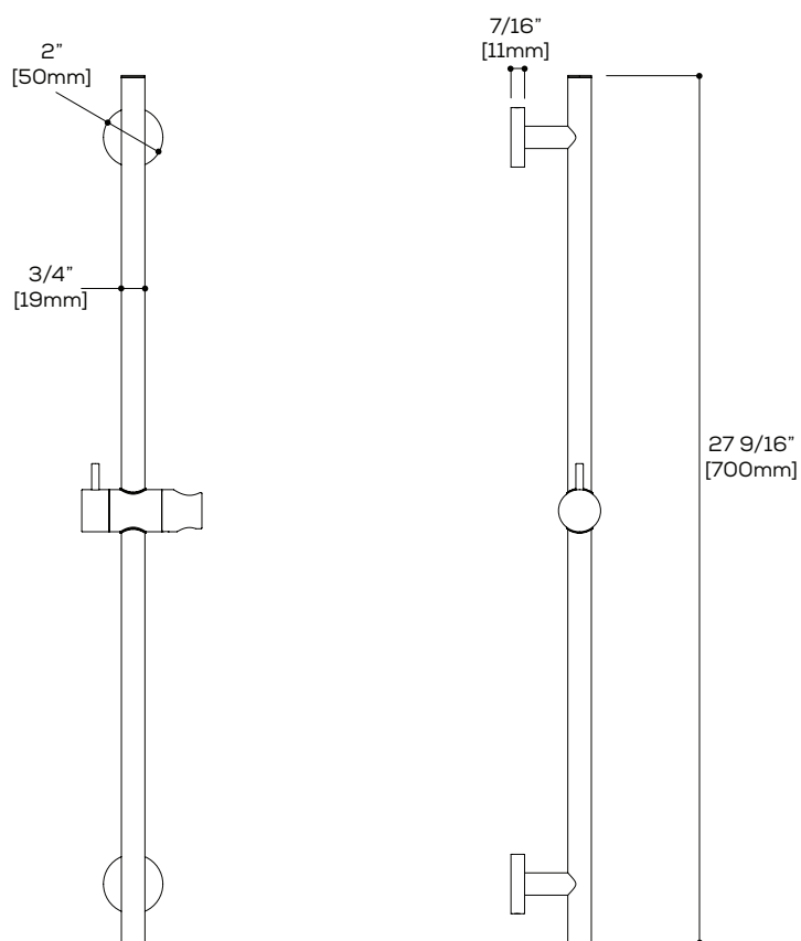
ABSPXPR80 Slider / Curseur
